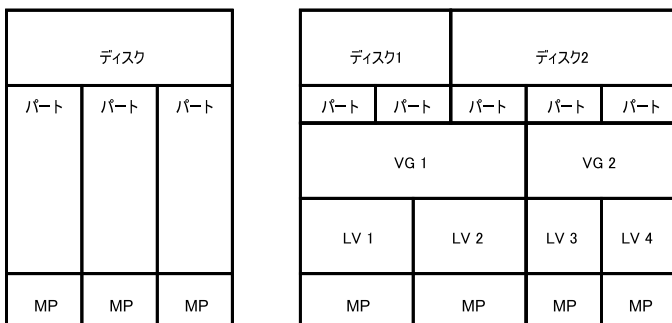
図 15.3 物理パーティショニング対LVM
